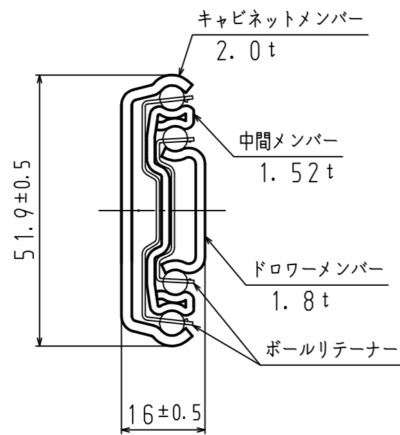
P矢視断面 (S: 1/1)
