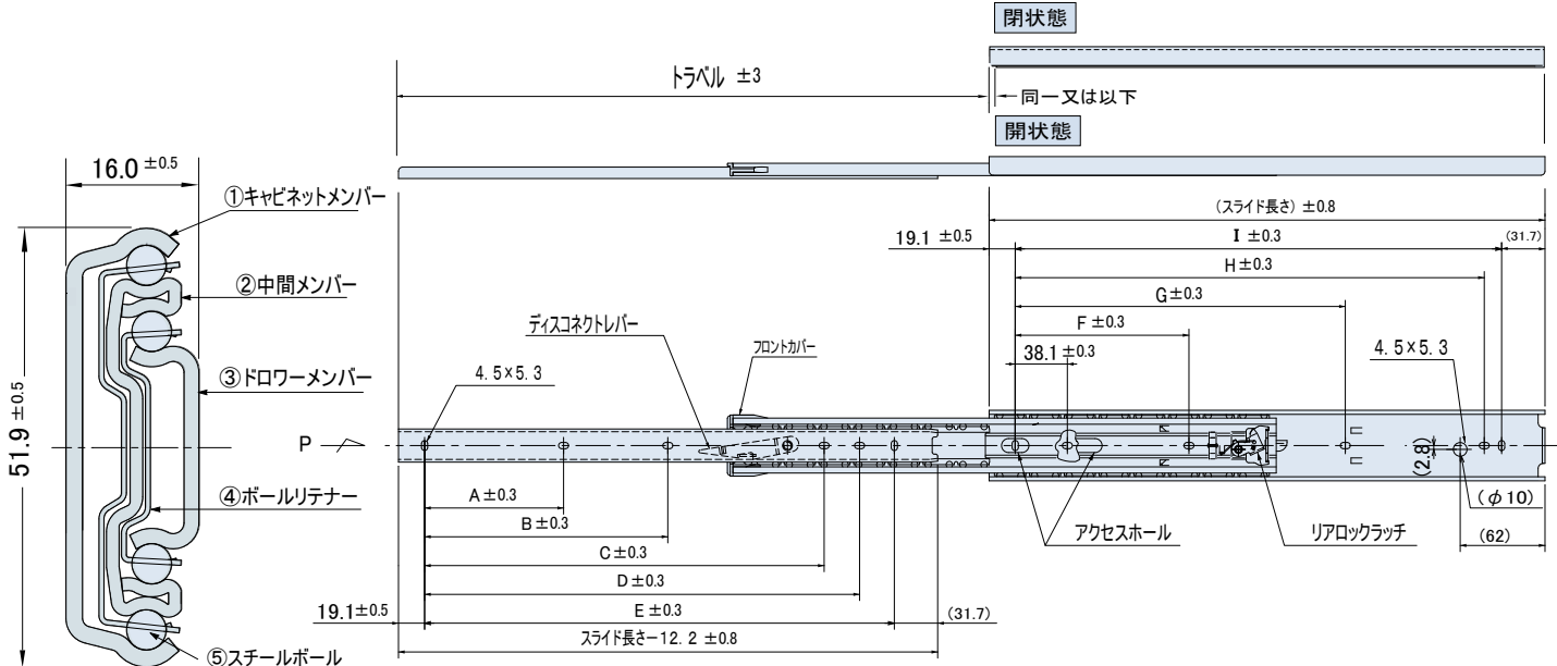
P矢視断面図 (S:1/1)
