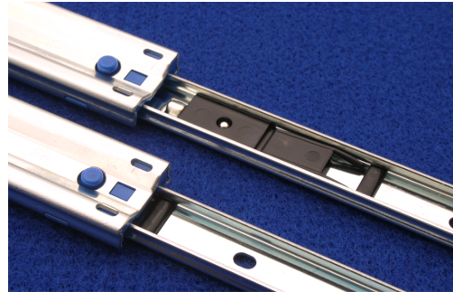
モデル3273SC ディスコネクトスプリング解除部拡大
